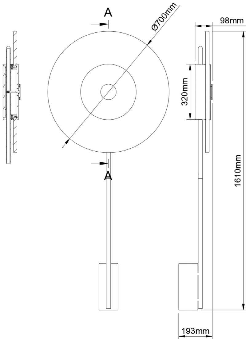
A-A (1: 10)
